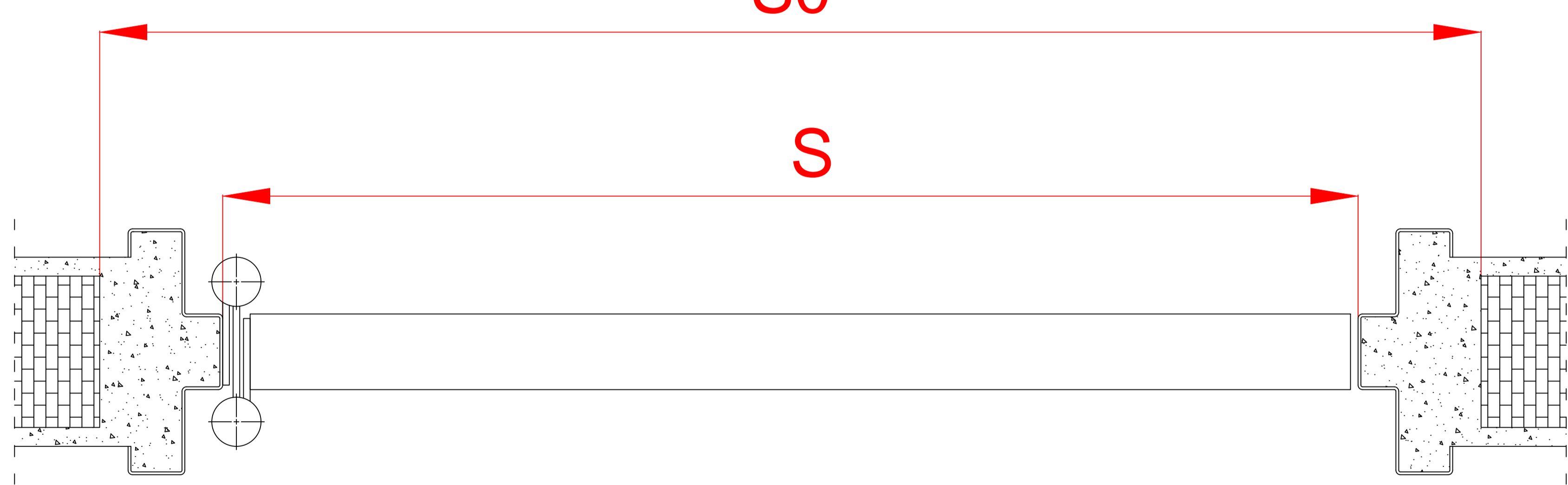
B-B (2:1)
