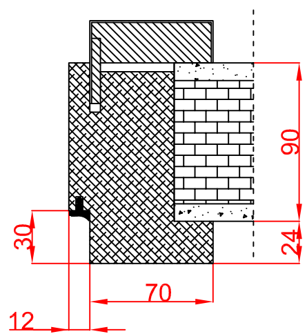
A-A (5:1)
